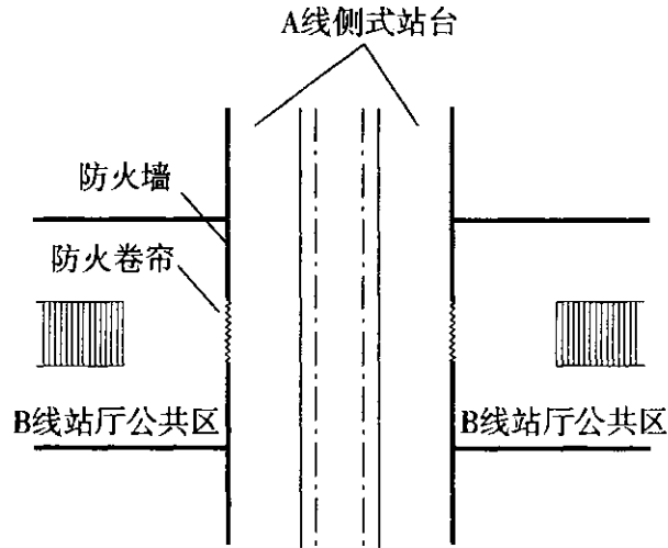
图9 侧式站台与同层站厅换乘防火隔离示意图
