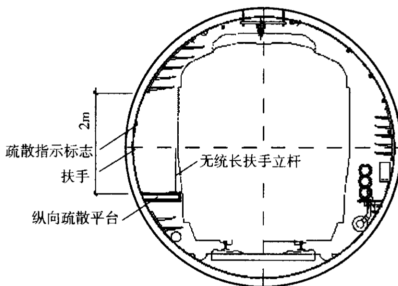
图 16 地下区间纵向疏散平台布置示意图
