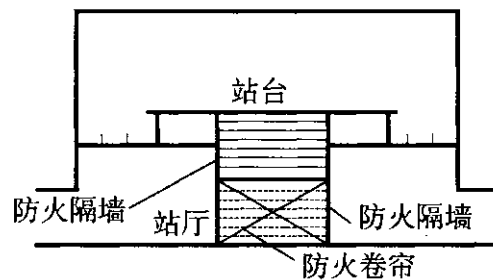
图 10 站厅层位于站台下方防火隔离示意图
