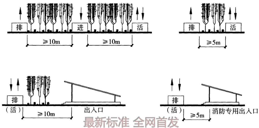
图1 各敞口低风井之间最小水平距离示意图
